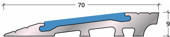
Elite Trim 7940
